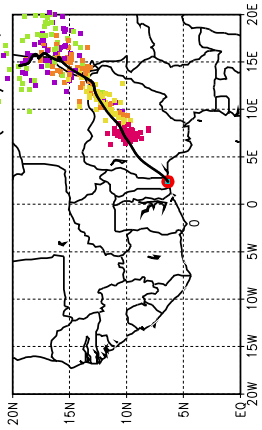
Ballons laches a J+96 h (06/07, 12 UTC)
