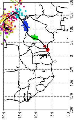
Ballons laches a J+18 h (03/07, 18 UTC)
