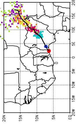
Ballons laches a J+66 h (06/07, 18 UTC)
