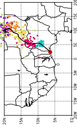
Ballons laches a J+78 h (13/07, 18 UTC)
