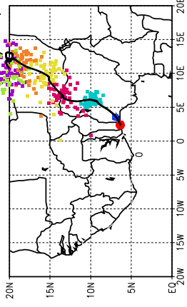
Ballons laches a J+66 h (13/07, 6 UTC)
