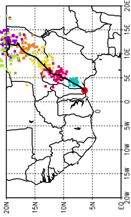
Ballons laches a J+84 h (14/07, 12 UTC)
