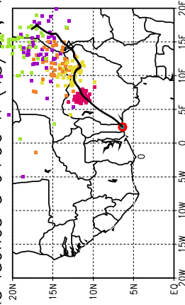
Ballons laches a J+96 h (18/07, 12 UTC)
