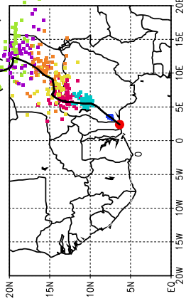
Ballons laches a J+66 h (24/07, 18 UTC)
