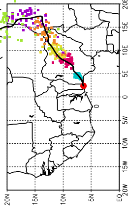
Ballons laches a J+78 h (27/07, 6 UTC)
