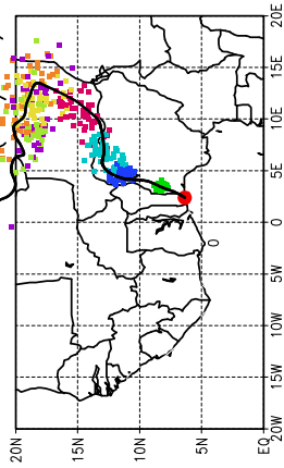
Ballons laches a J+36 h (25/07, 12 UTC)
