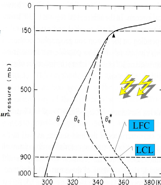
Situation convective typique en région tropicale
